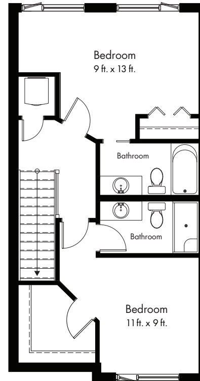
Upper Floor: 633 S.F.
